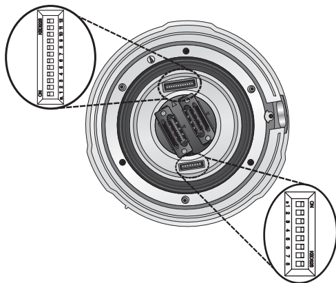
DIP переключатель ID камеры (SW1)в
